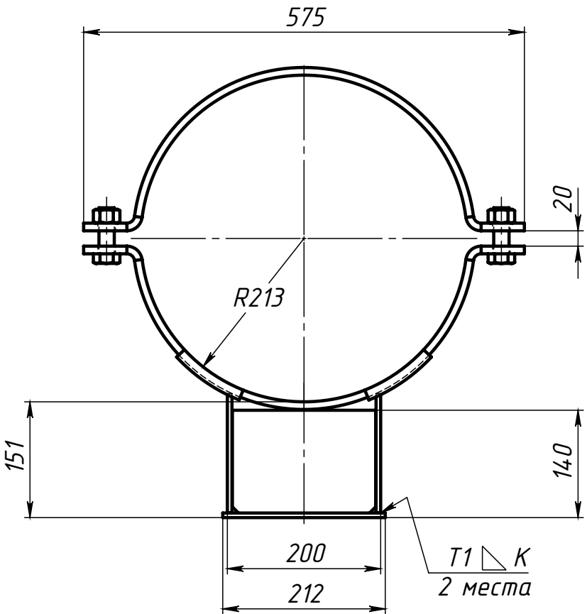
Поз.4 (Полухомут)
