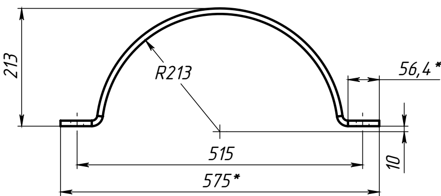
Поз.4 (Полухомут)
